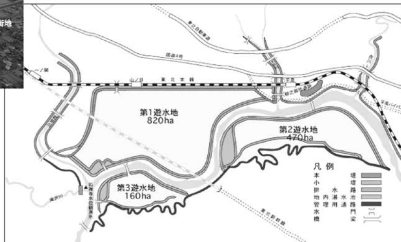
【一関遊水地 計画概要図】
